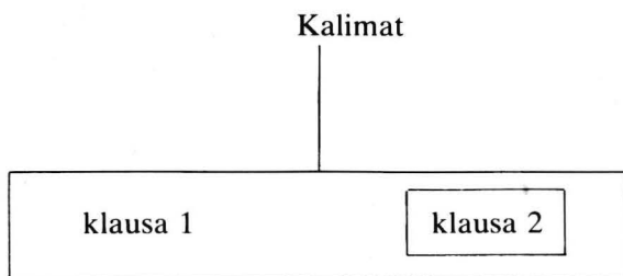
Bagan 10.2: Subordinasi
