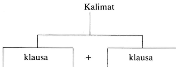
Bagan 10.1: Koordinasi
