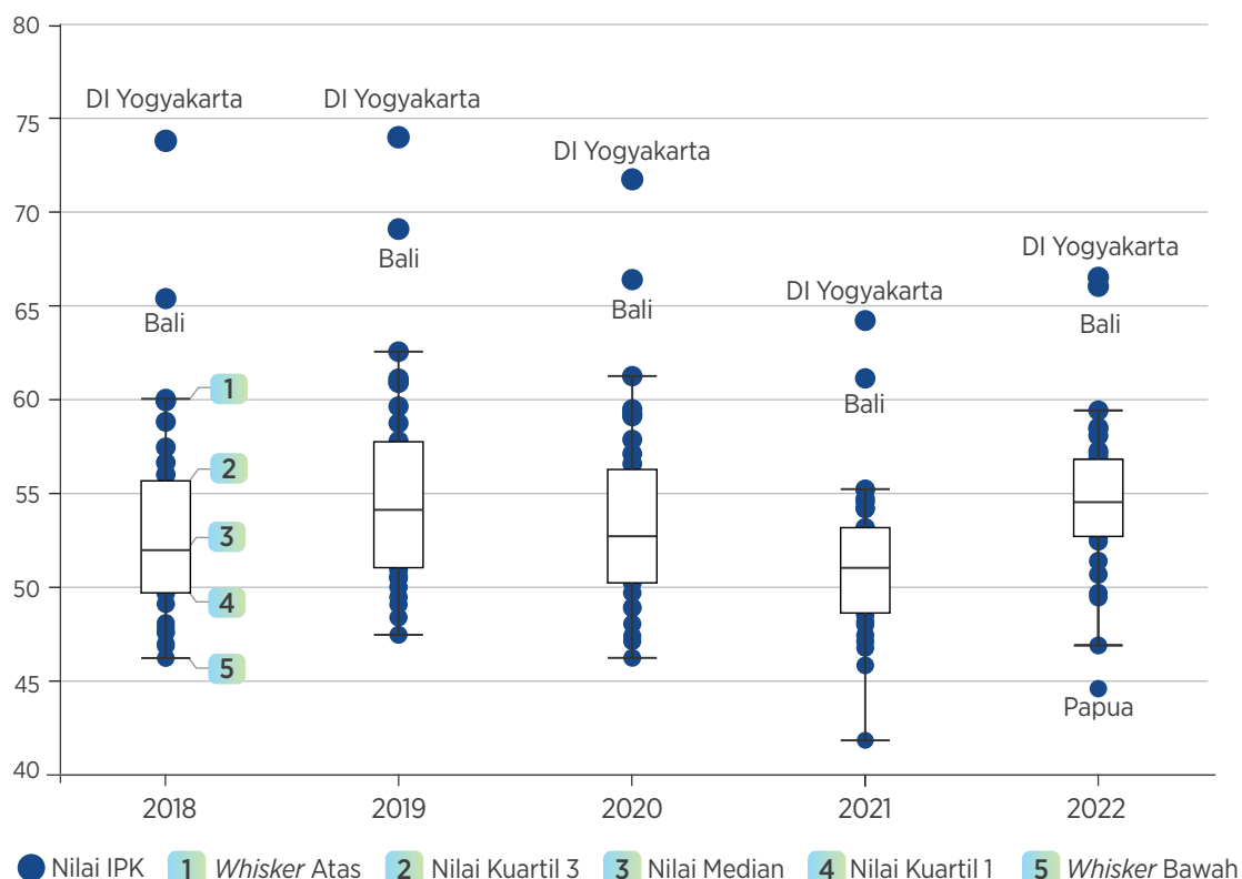
Grafik Distribusi IPK Provinsi
