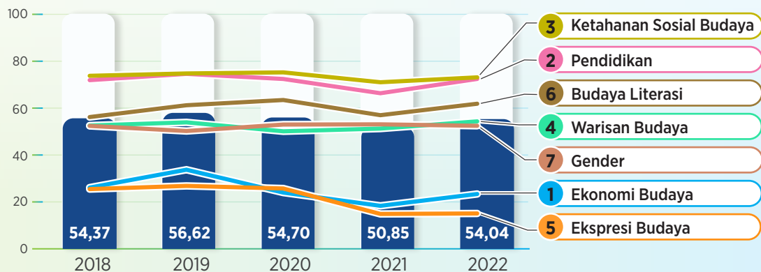
IPK Kepulauan Bangka Belitung dan Dimensi Pembentuk 2018-2022
