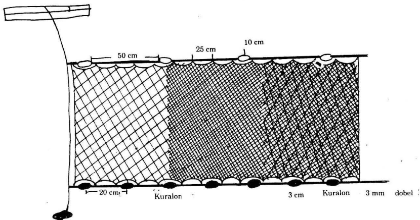
gambar 3.10 Alat tangkap Trammel net
